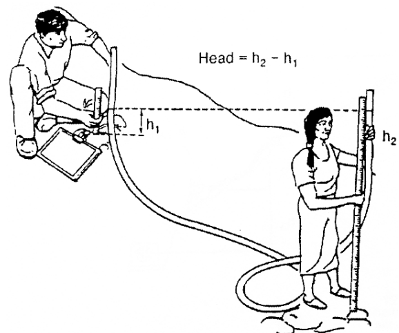
vervalmeting met een waterslang en een meetlat
